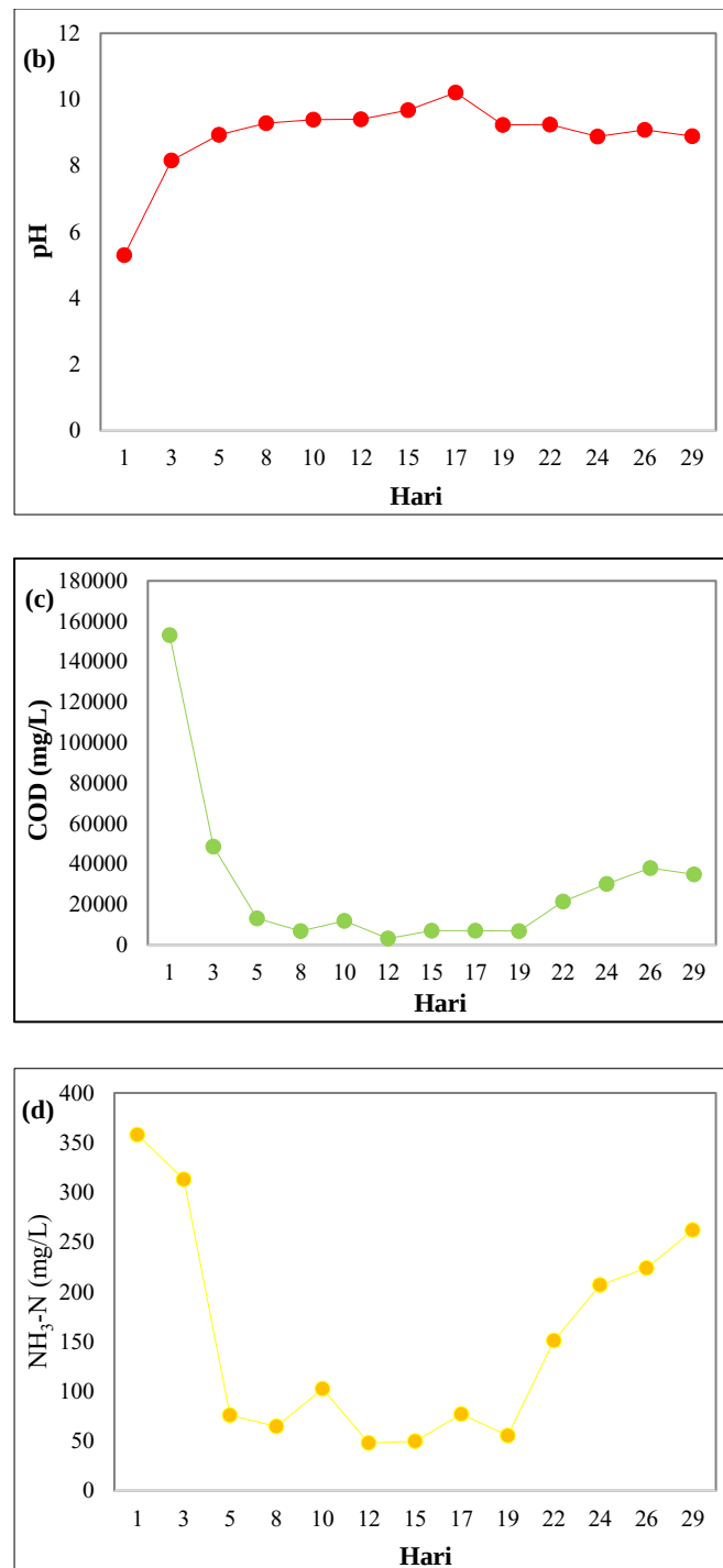
Rajah 2. Bacaan parameter diambil semasa proses penyesuaian iklim bakteria selama 4 minggu berturut-turut (a) suhu (b) pH (c) COD (d) NH 3 -N
