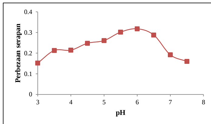
Rajah 3. Kesan pH terhadap rangsangan sensor apabila ditindak balas dengan ion \text{Al}^{3+} . Keadaan eksperimen: [\text{Al}^{3+}] = 7.41 \times 10^{-5} \text{ mol L}^{-1}
