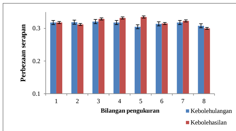
Rajah 7. Kajian kebolehhulangan dan kebolehasilan sensor terhadap ion \text{Al}^{3+} berkepekatan 7.41 \times 10^{-5} \text{ mol L}^{-1}
