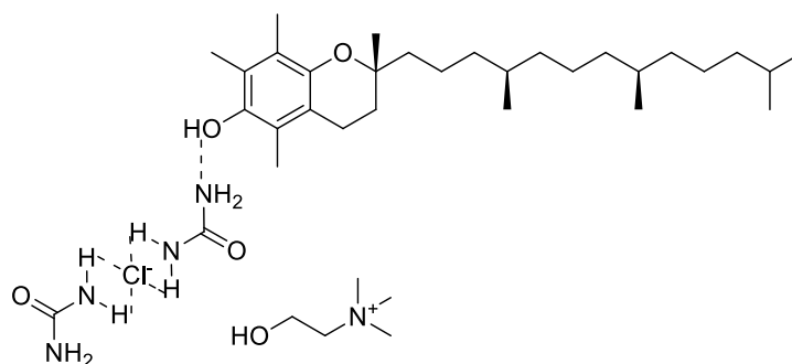
Rajah 9. Analog ikatan hidrogen yang terhasil antara sebatian \alpha -T dan DES relina yang dirujuk daripada kajian Xiaolei et al [25]
