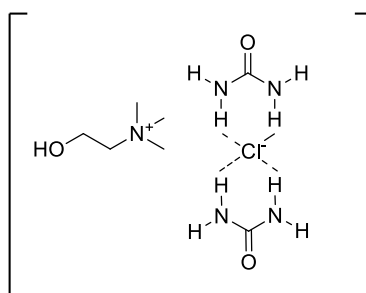
Rajah 3. Ikatan hidrogen yang terbentuk dalam struktur DES relina
