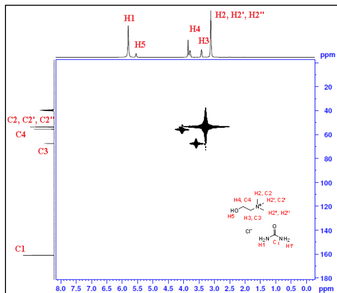
Rajah 6. Spektrum HMQC bagi DES relina
