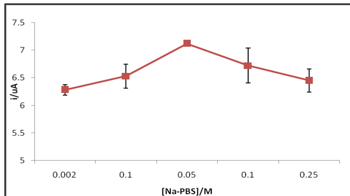
Rajah 9. Kesan kepekatan penimbal terhadap penghibridan DNA. Penghibridan dilakukan dalam pelbagai kepekatan penimbal Na-fosfat pH 7.0 yang mengandungi 1.5 M NaCl dan 30 \mu\text{M} [\text{Ru}(\text{bpy})_2\text{PIP}]^{2+}
