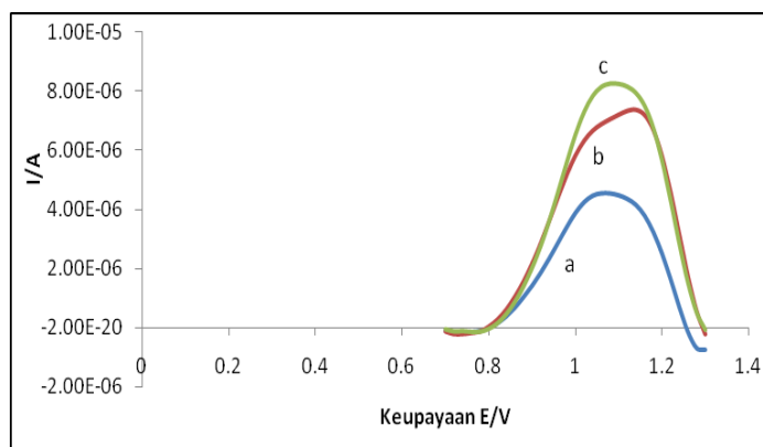
Rajah 4. Voltammogram pembezaan denyutan (DPV) bagi interaksi antara [\text{Ru}(\text{bpy})_2\text{PIP}]^{2+} dengan a) prob DNA sahaja (bebenang tunggal), b) DNA bukan sasaran selepas penghibridan dan c) DNA sasaran selepas penghibridan
